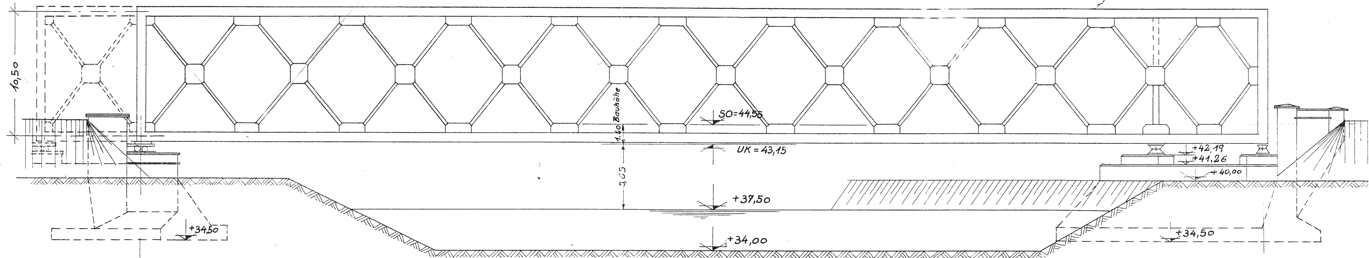
Ansicht von Osten M=1:200
