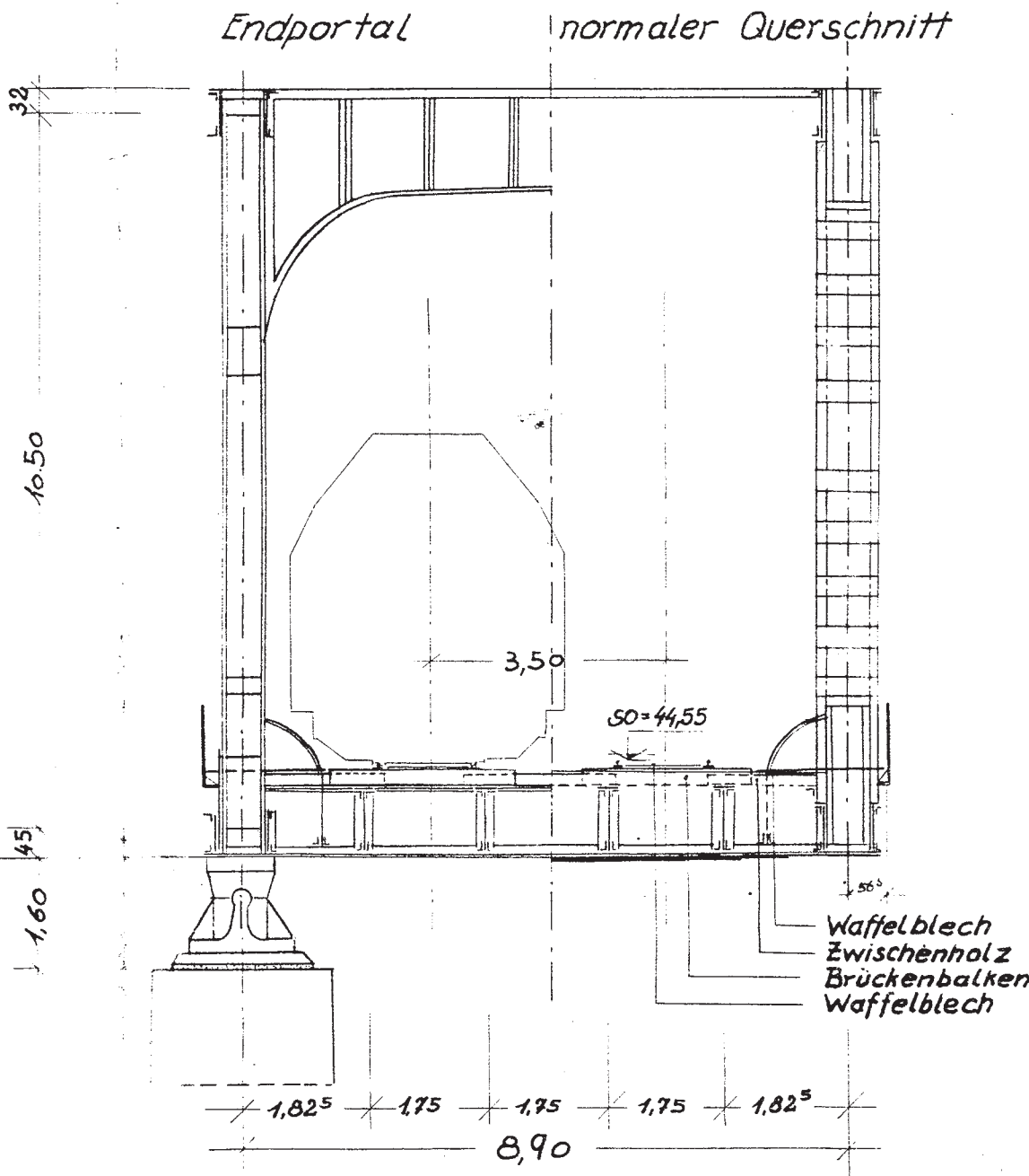
Querschnitt M=1:100
